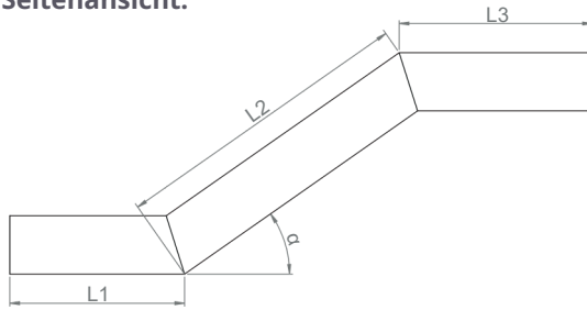
Seitenansicht:
